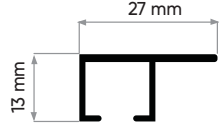
NL 2015 - Beyaz/Siyah Yandan Çıkmalı Tekli Ray
