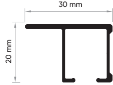
NL 2001 - Beyaz/Siyah Bilyalı Rulmanlı Tekli Ray
