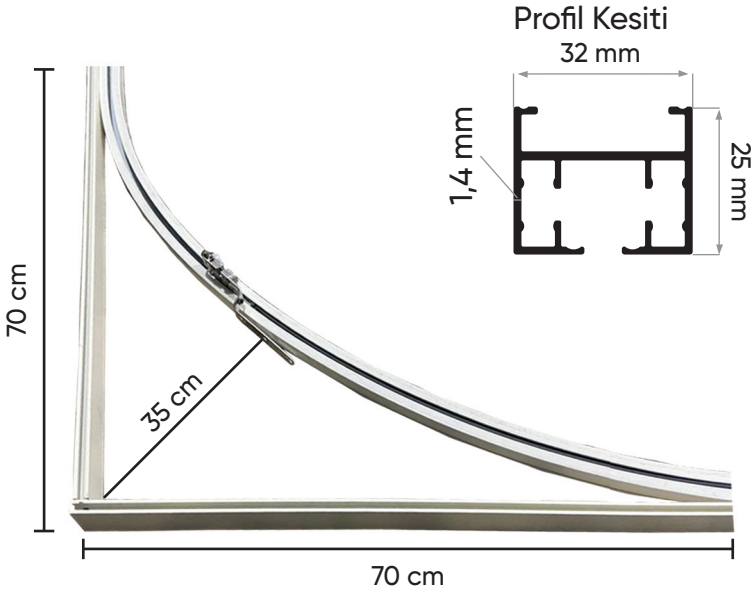
NL 17001 Oval Büküm
